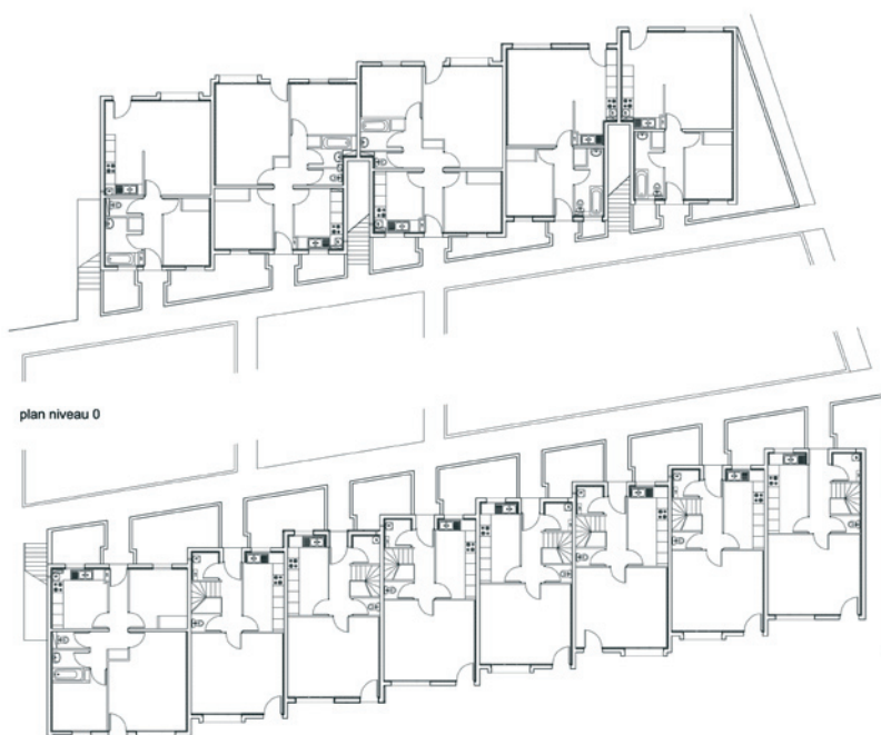
Plan niveau rez-de-chaussée © PO&PO
